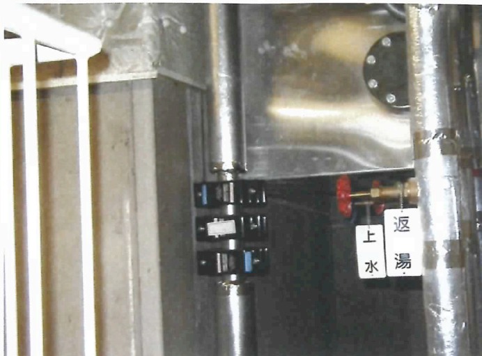
わかば寮（5階建）赤水対策でマグネタイザーM2*3set 取付 H14.7.15 50A 給水管に採用。約1ヶ月で赤水解消。1階に保育所があり乳幼児のミルクもこの水で作られており、赤水の再発もなく磁気水の様々なメリットを楽しんでおられます。
